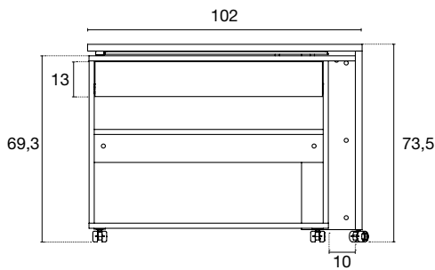
Position fermée
